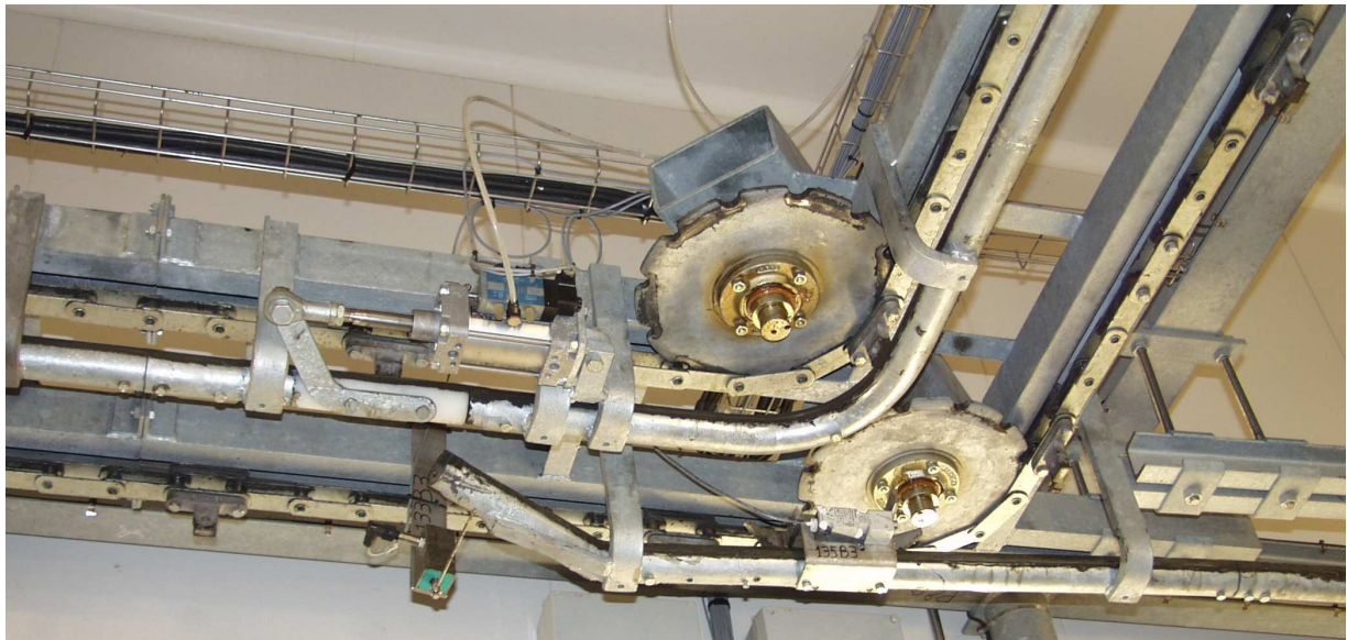
Convoyeurs de réfrigération
