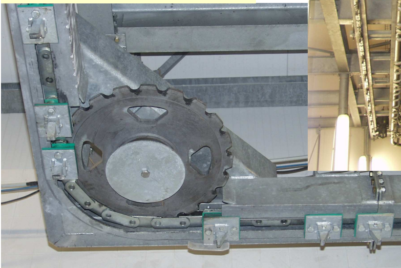
Roue de détour convoyeur d'habillage
