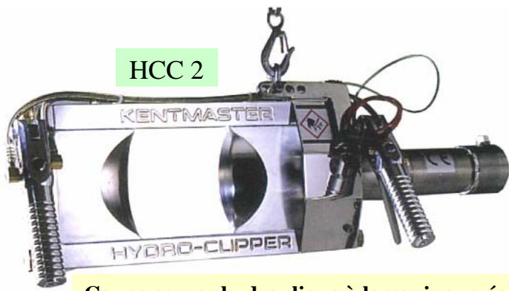
Coupe cornes hydraulique à lames incurvée
